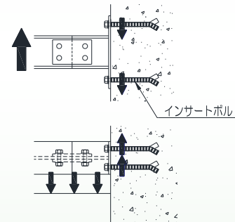
耐風梁使用例
